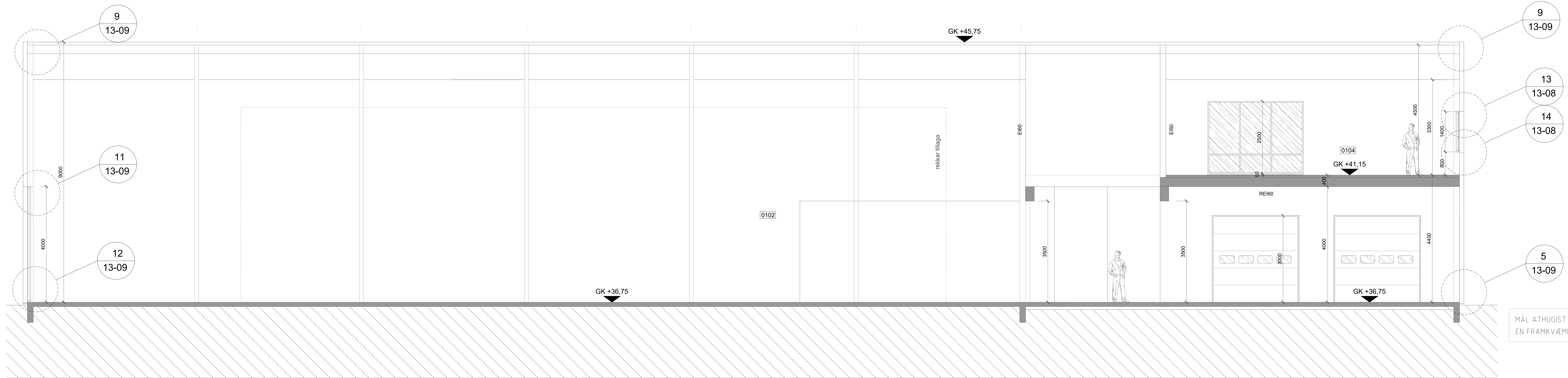
sneiðing 5-5
