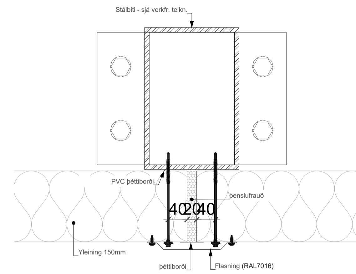
DEILI 5 - 13-01
