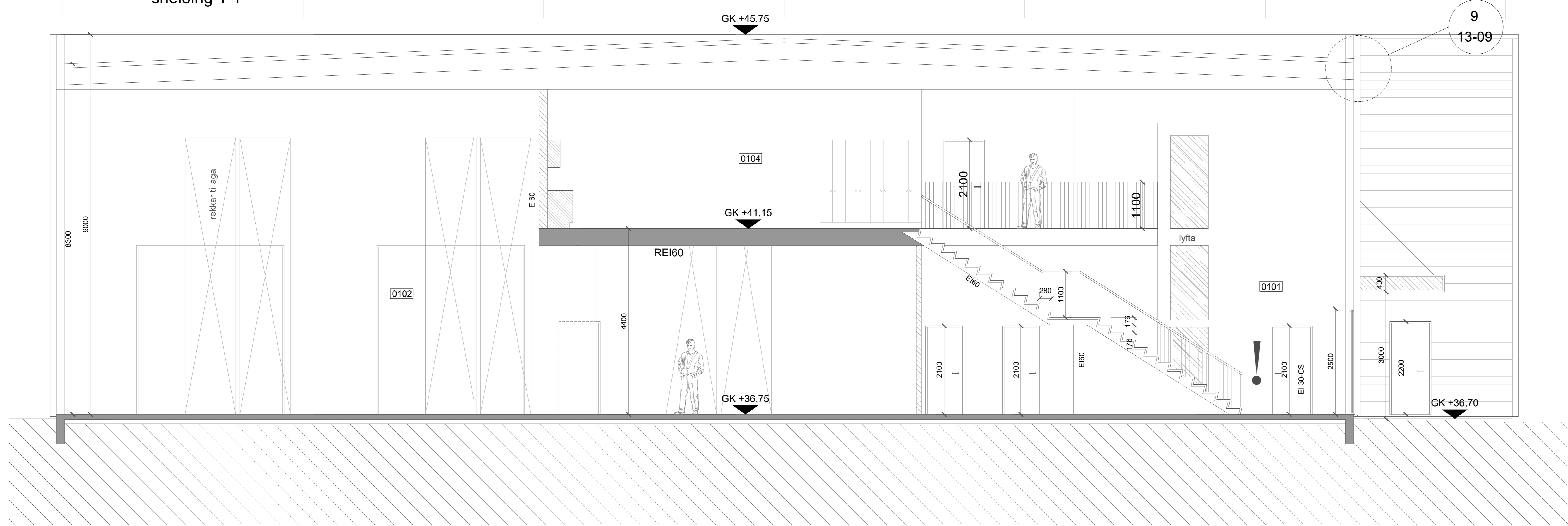
sneiðing 2-2
