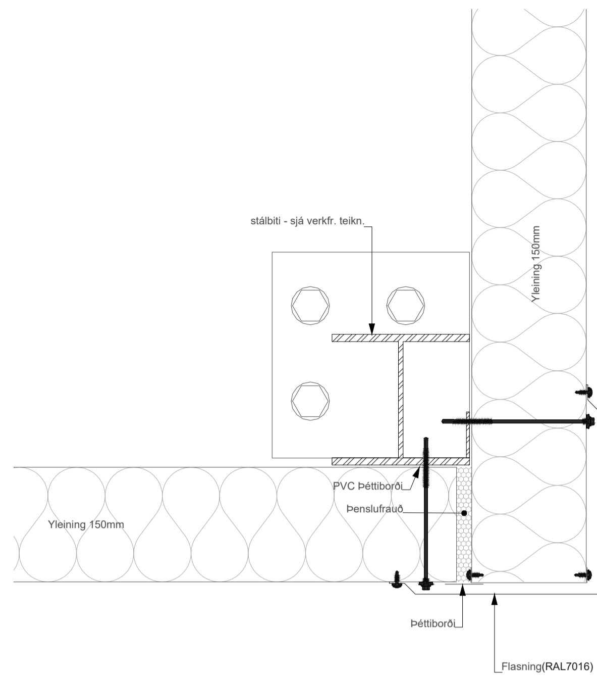
DEILI 1 - 13-01
