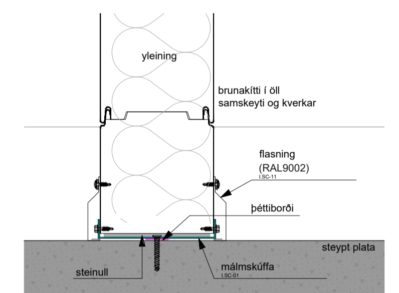
DEILI 21 - 13-01
