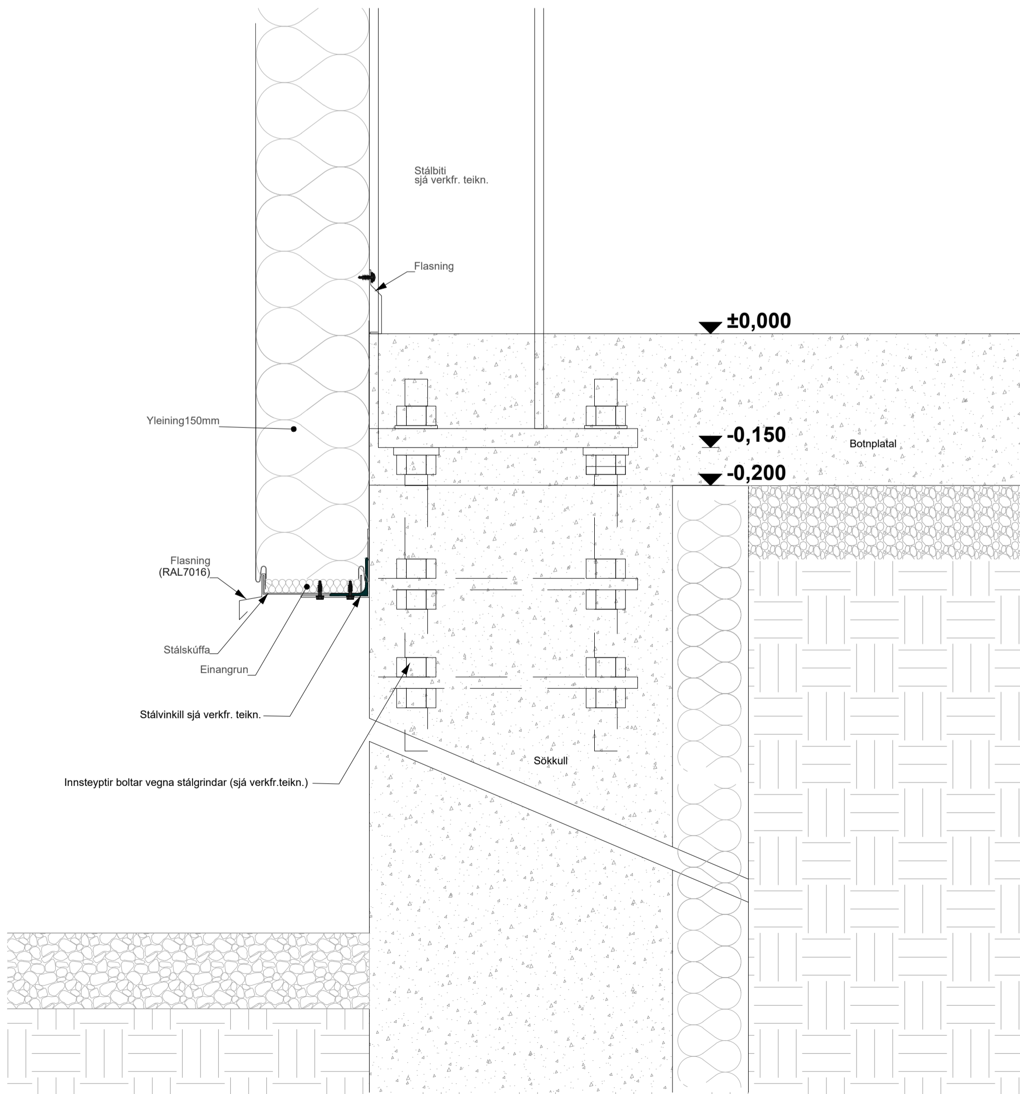
DEILI 19 - 13-05
