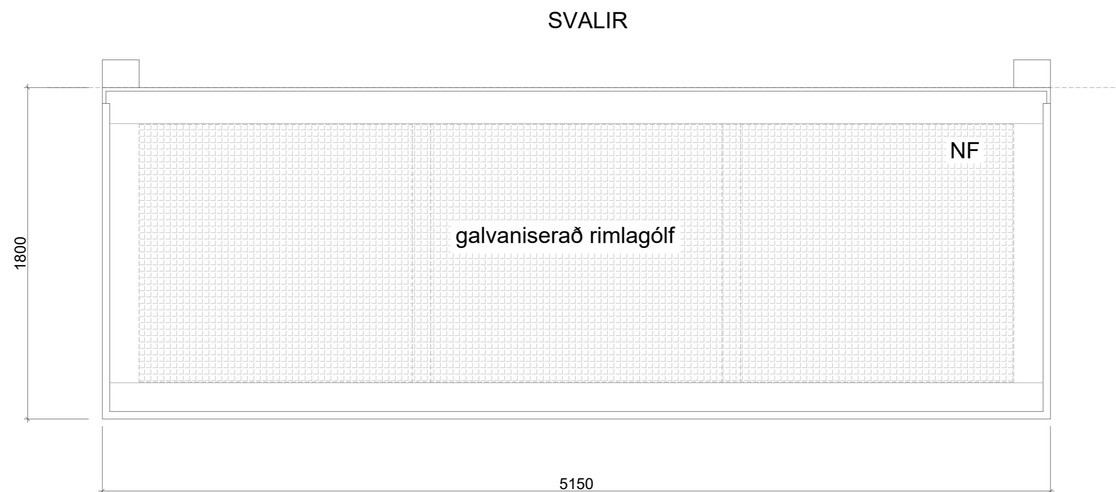
GRUNNMYND
