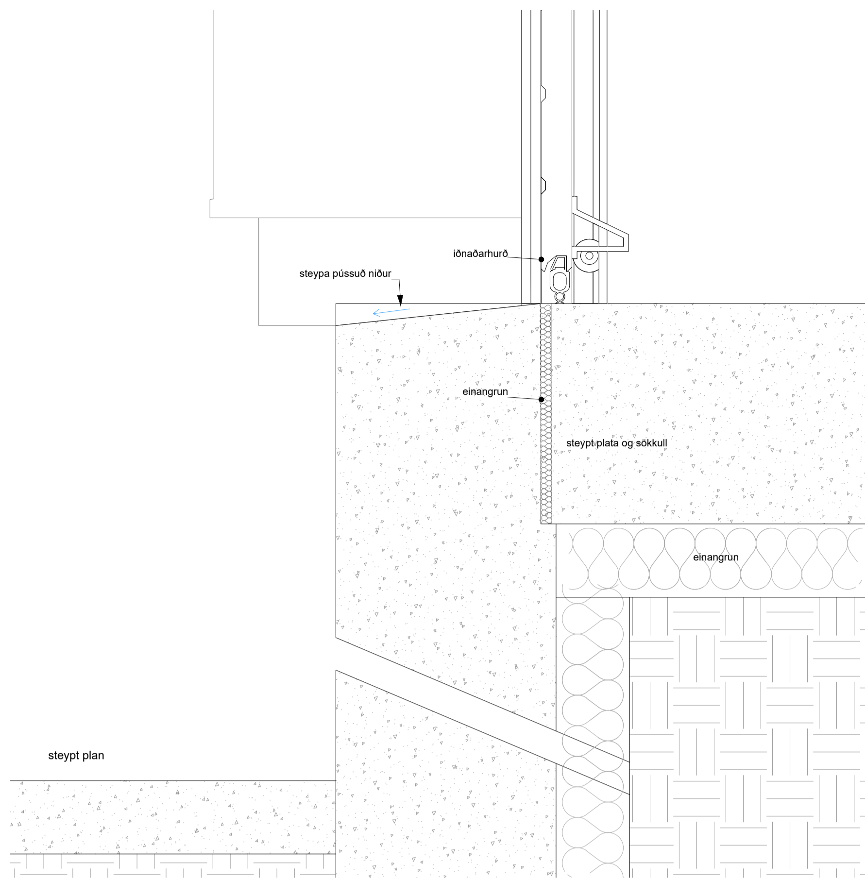
DEILI 18 - 13-05
