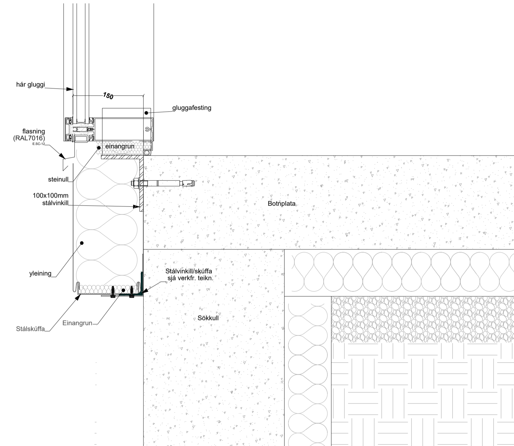
DEILI 17 - 13-07/13-08
