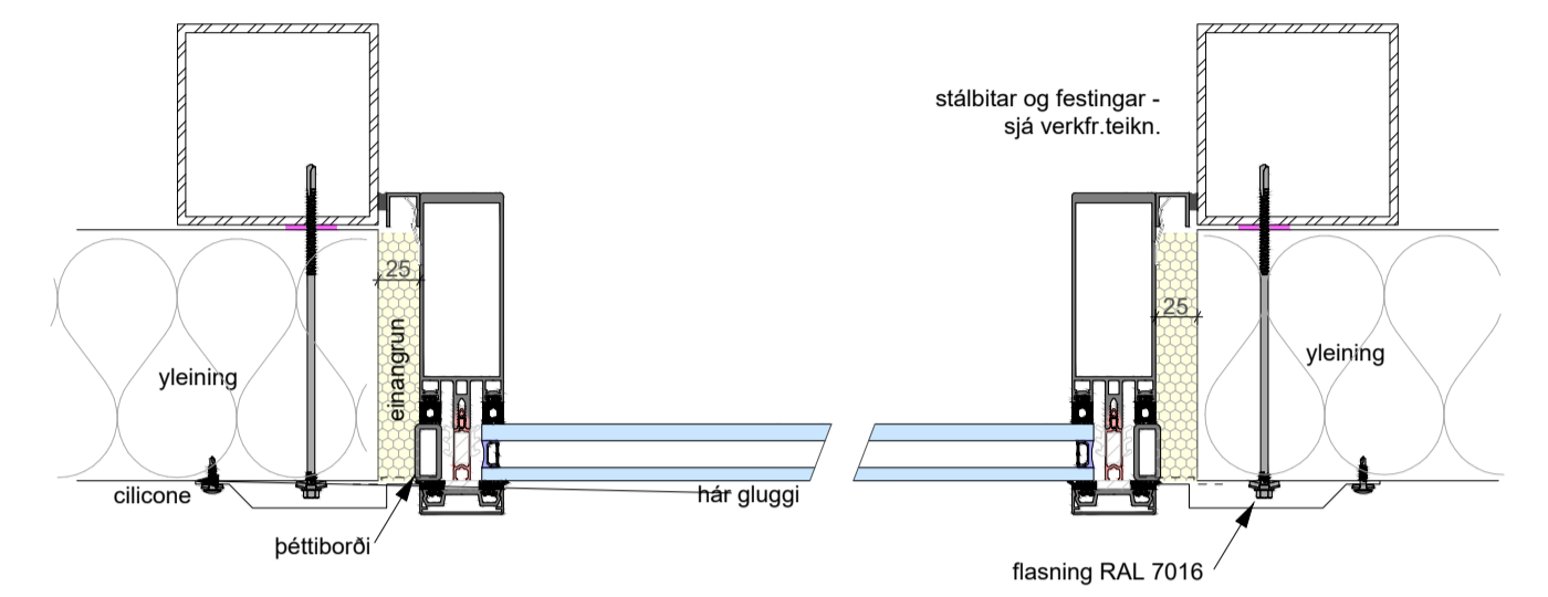
DEILI 20 - 13-01
