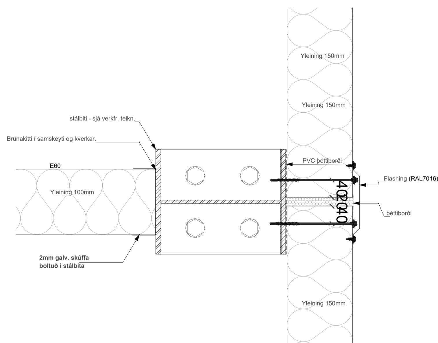
DEILI 6 - 13-01
