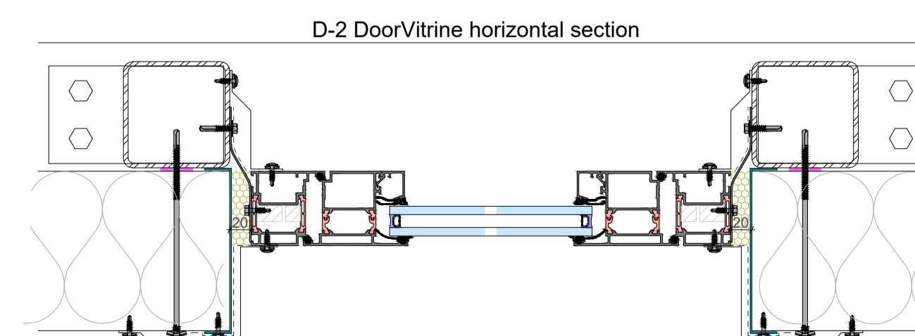
DEILI 4 - 13-01
