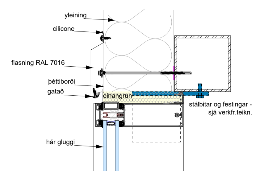
DEILI 16 - 13-06
